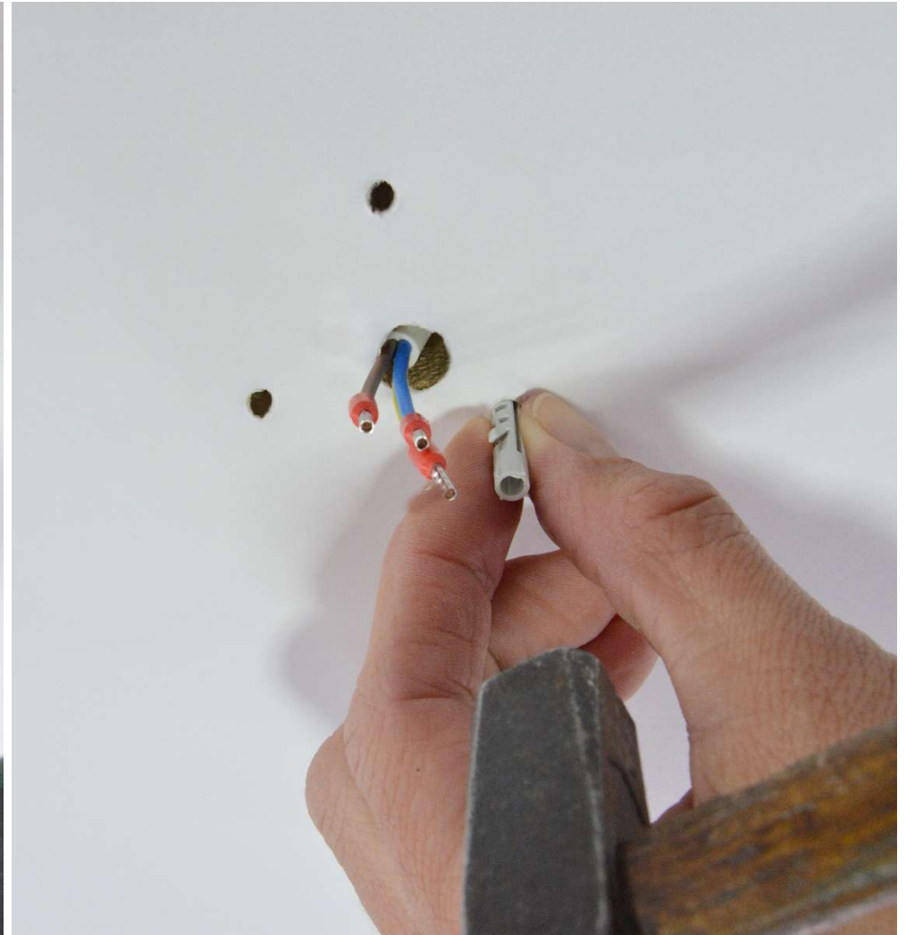
04. setzen Sie die mitgelieferten Dübel ein.
